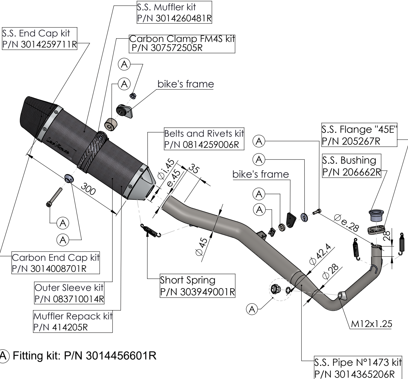
dB-Killer n°62 P/N 3014259802R
