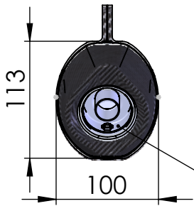
dB-Killer n°62 P/N 3014259802R
